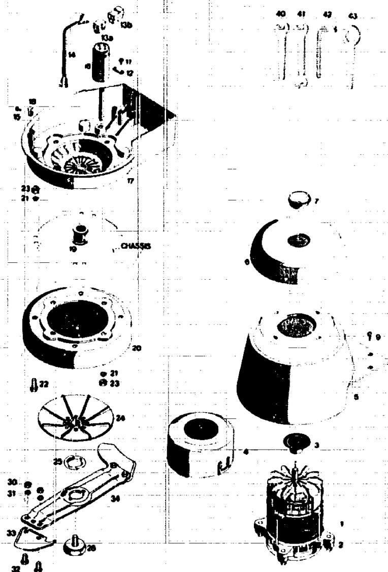
Motor mit Messerbalken
