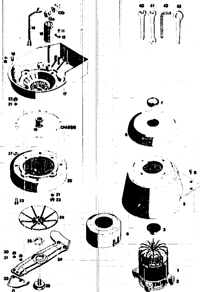
Motor mit Messerbalken
