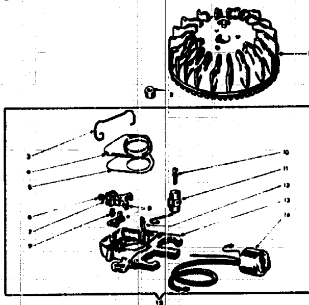
Ersatzteile Zündanlage
