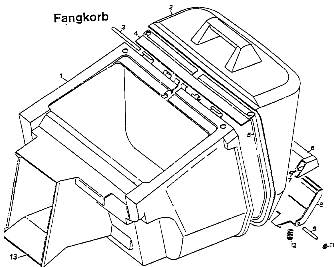
Fangkorb
