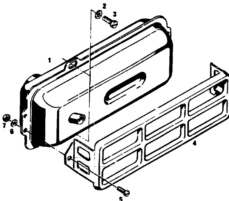
Auspufftopf
