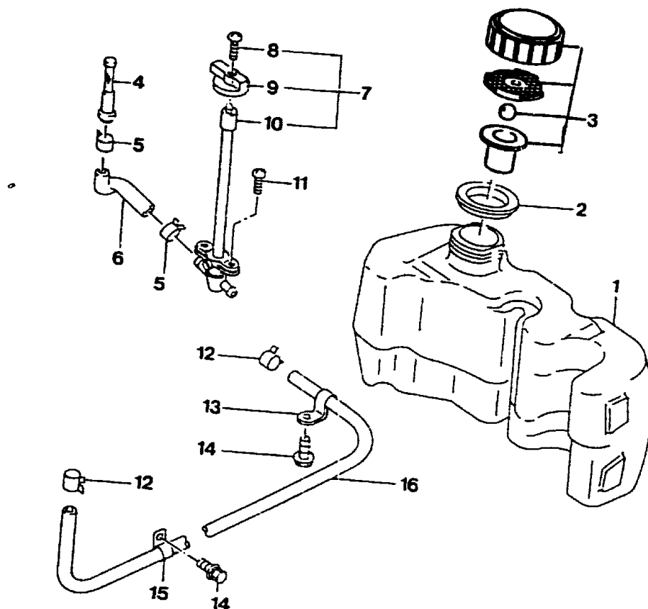
Tank FC 150 V - ES 63, ES 64
