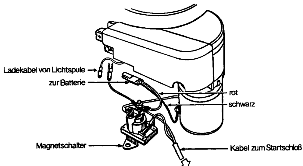
Verkabelungsplan
